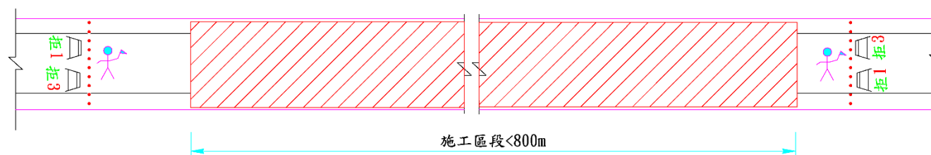
AC鋪道路封閉改道交通維持示意圖
