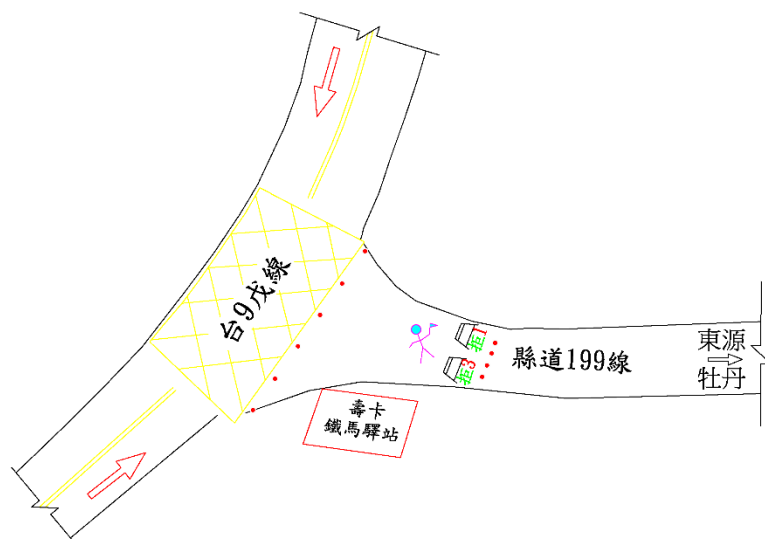
封閉道路交通維持示意圖(台9戊線與199線路口)
