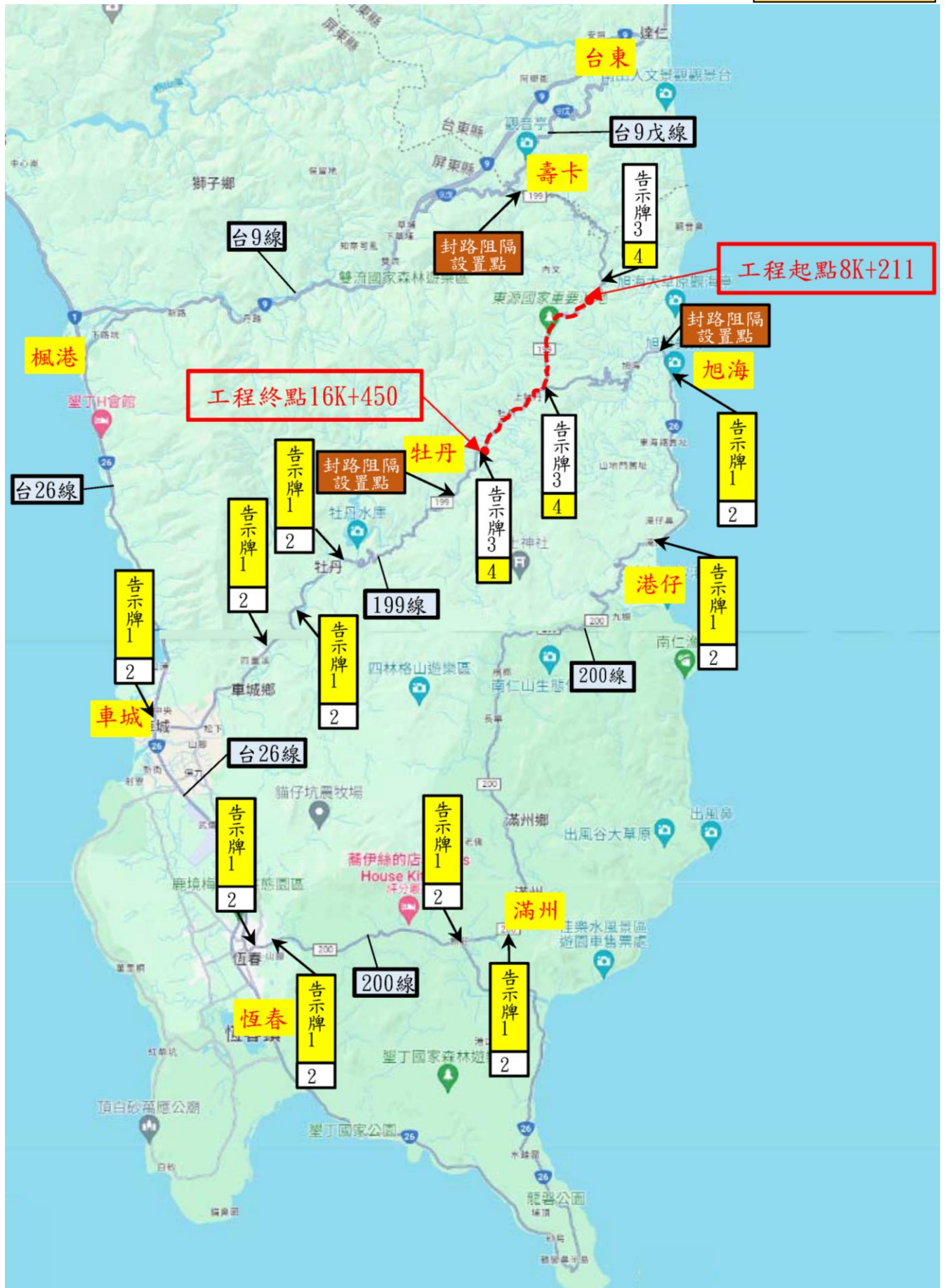
道路封閉施工、替代道路路線圖及開放通車時段等告示牌配置圖
