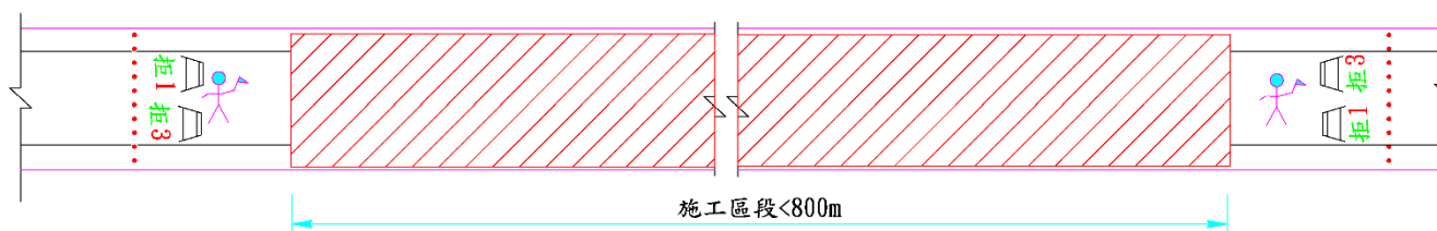
AC刨鋪道路封閉改道交通維持示意圖
